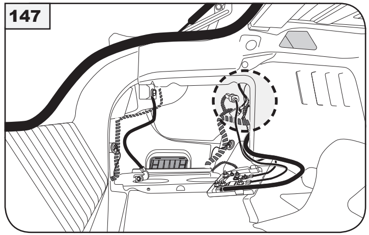
Sicherungskasten fusebox
