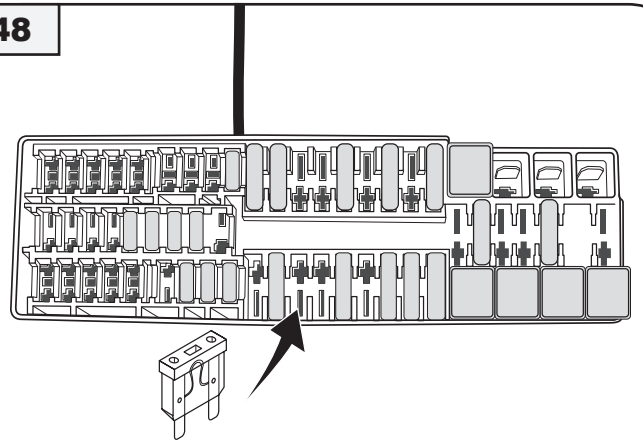
Sicherung Kasten Fusebox
