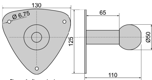
Figura 1: dimensioni
