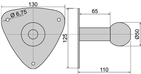
Bild 1: Dimensionen
